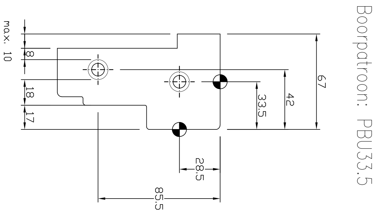
Maximale uitspraving bij standaard BU–boorpatroon sponing 17mm
