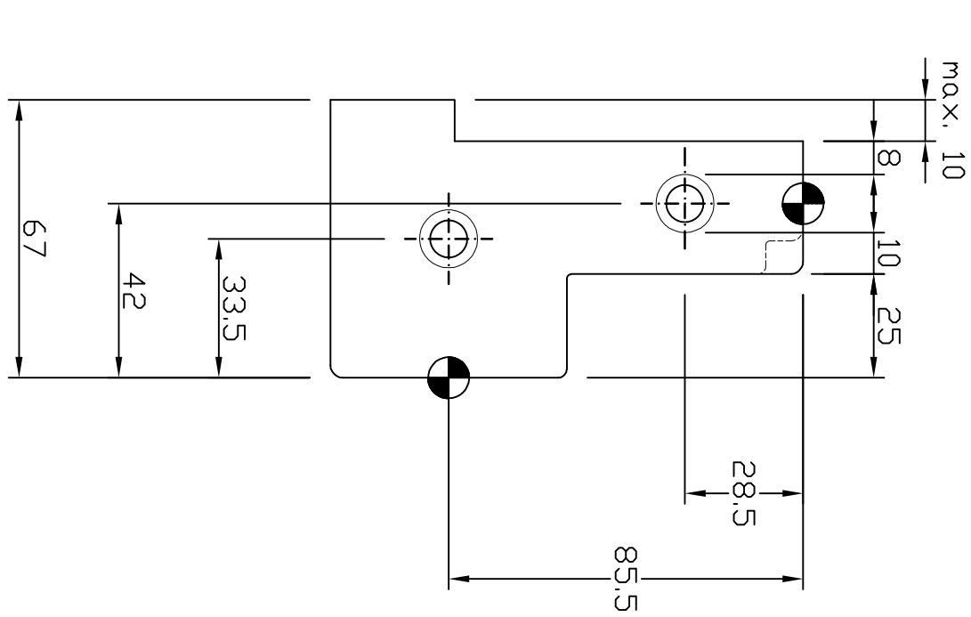
Maximale uitspraving bij standaard BI–boorpatroon sponing 25mm
