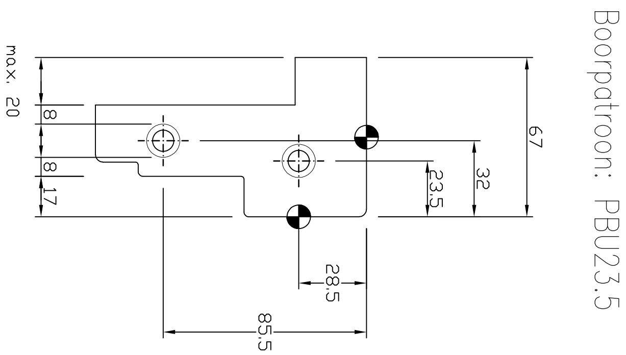
Maximale uitspraving bij aangepast BU–boorpatroon sponing 17mm
