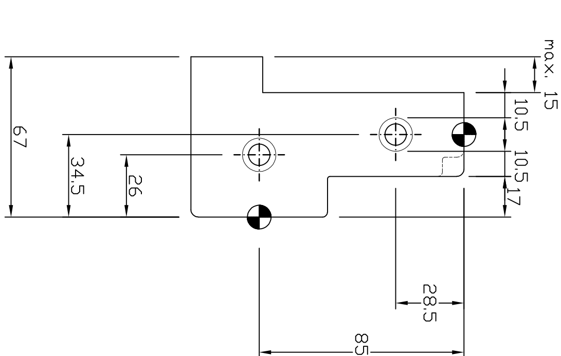
Aangepast BI–boorpatroon sponing 17mm bij uitspraving >10mm tot max. 15mm
