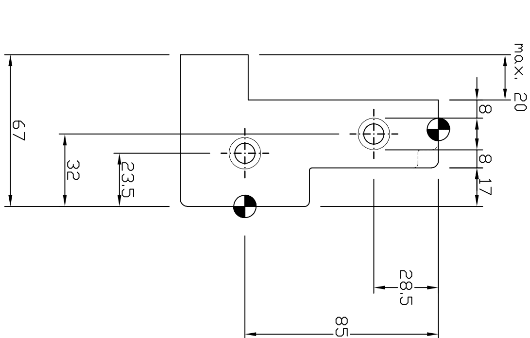
Maximale uitspraving bij aangepast BI–boorpatroon sponing 17mm
