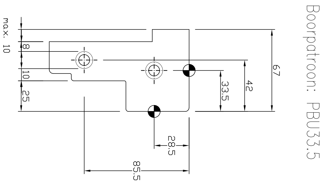
Maximale uitspraving bij standaard BU–boorpatroon sponing 25mm
