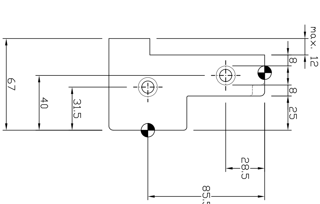
Maximale uitspraving bij aangepast BI–boorpatroon sponing 25mm
