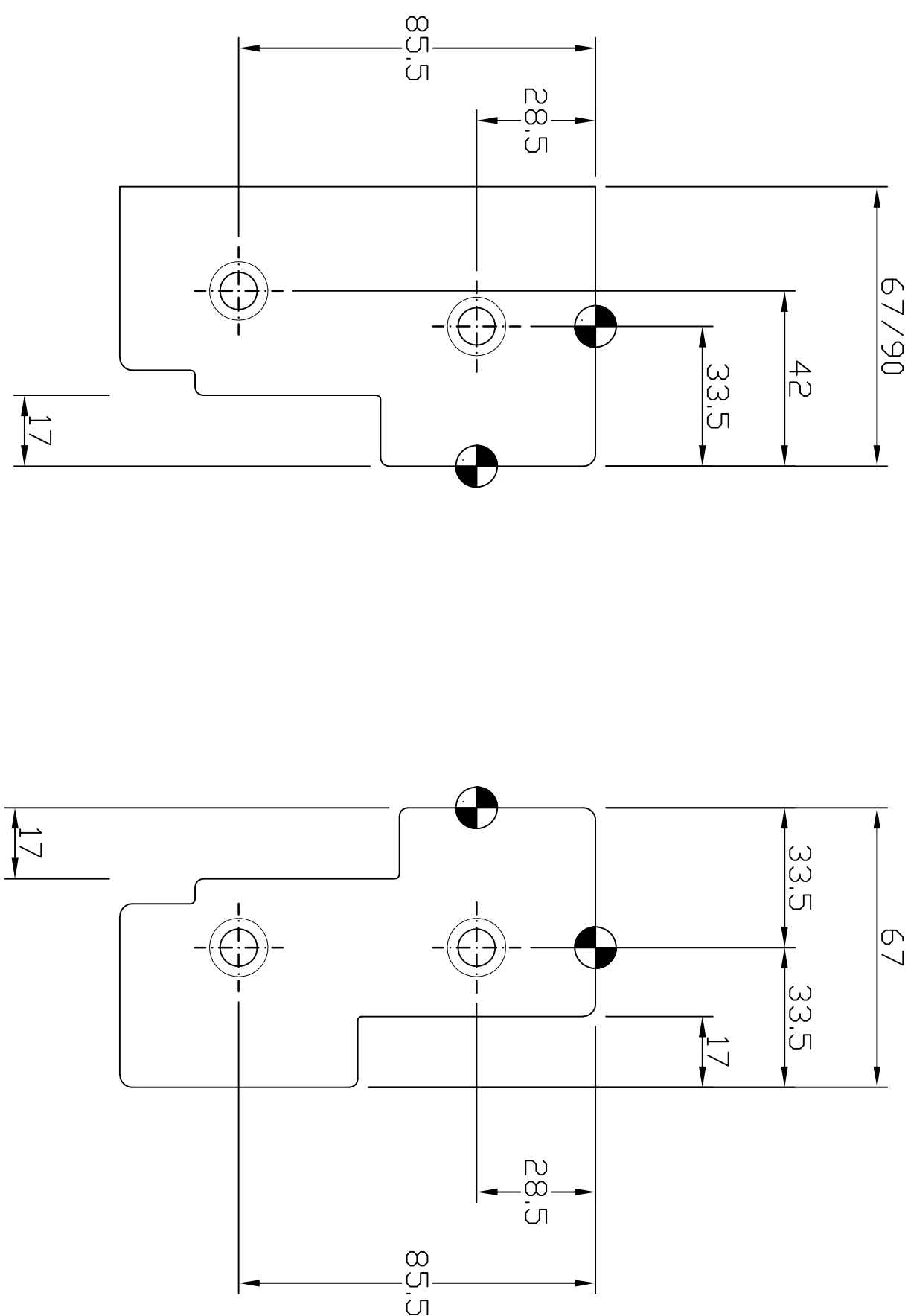
Boorpatroon: PBU33.5 Boorpatroon: PTNWS
