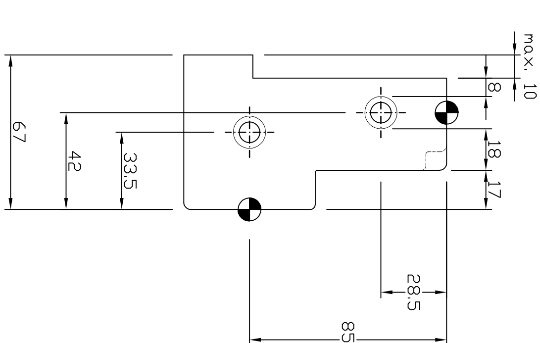
Maximale uitspraving bij standaard BI–boorpatroon sponing 17mm
