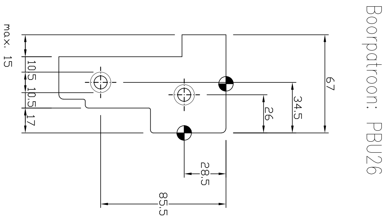
Aangepast BU–boorpatroon sponing 17mm bij uitspraving >10mm tot max. 15mm
