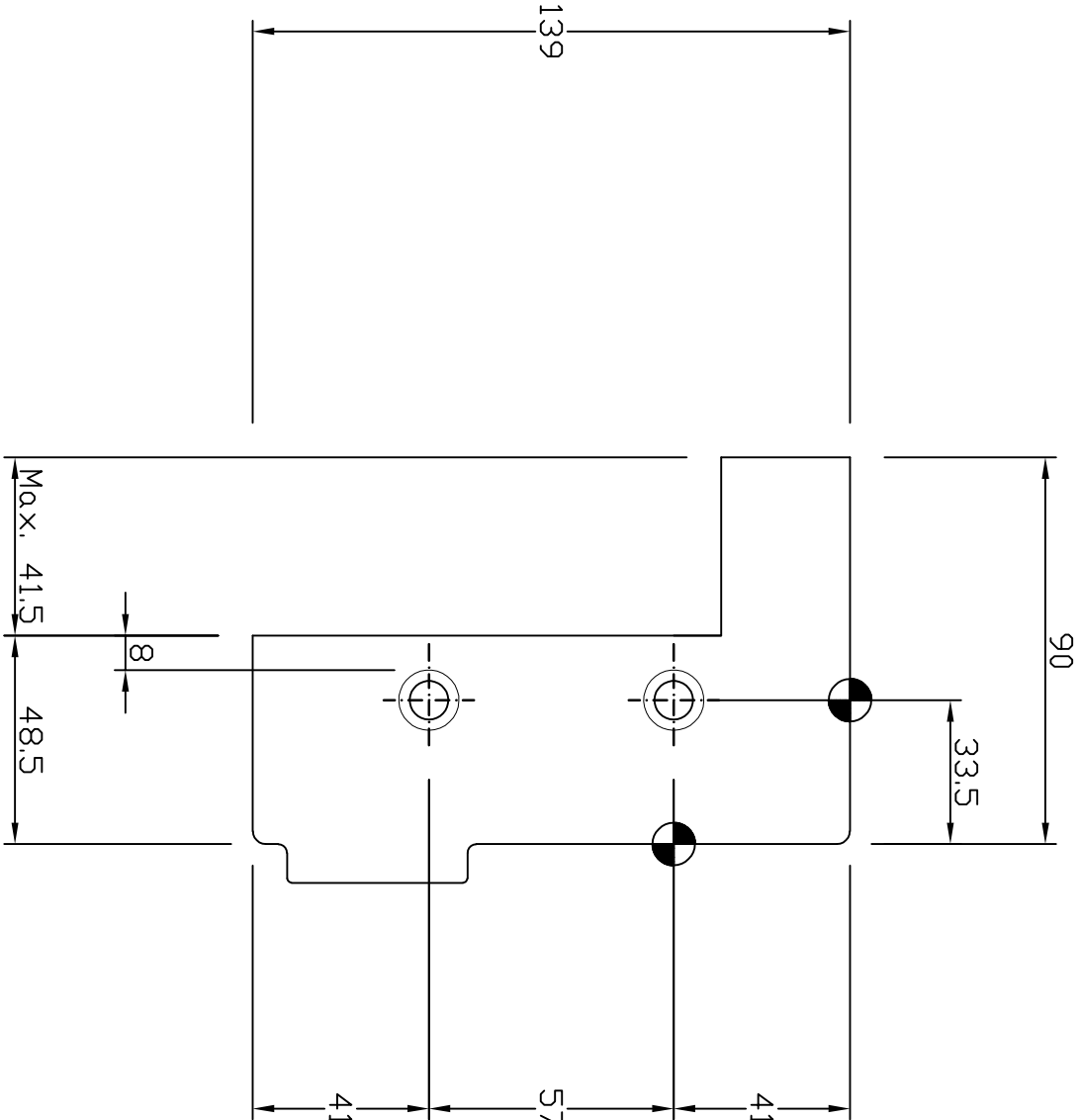
Boorpatroon: HFS33.5 (V139)
