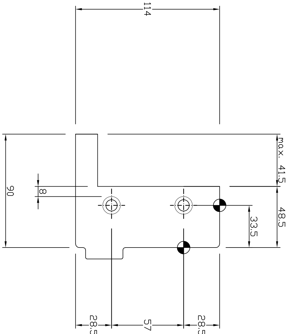
Boorpatroon: HFS33.5 (V114)
