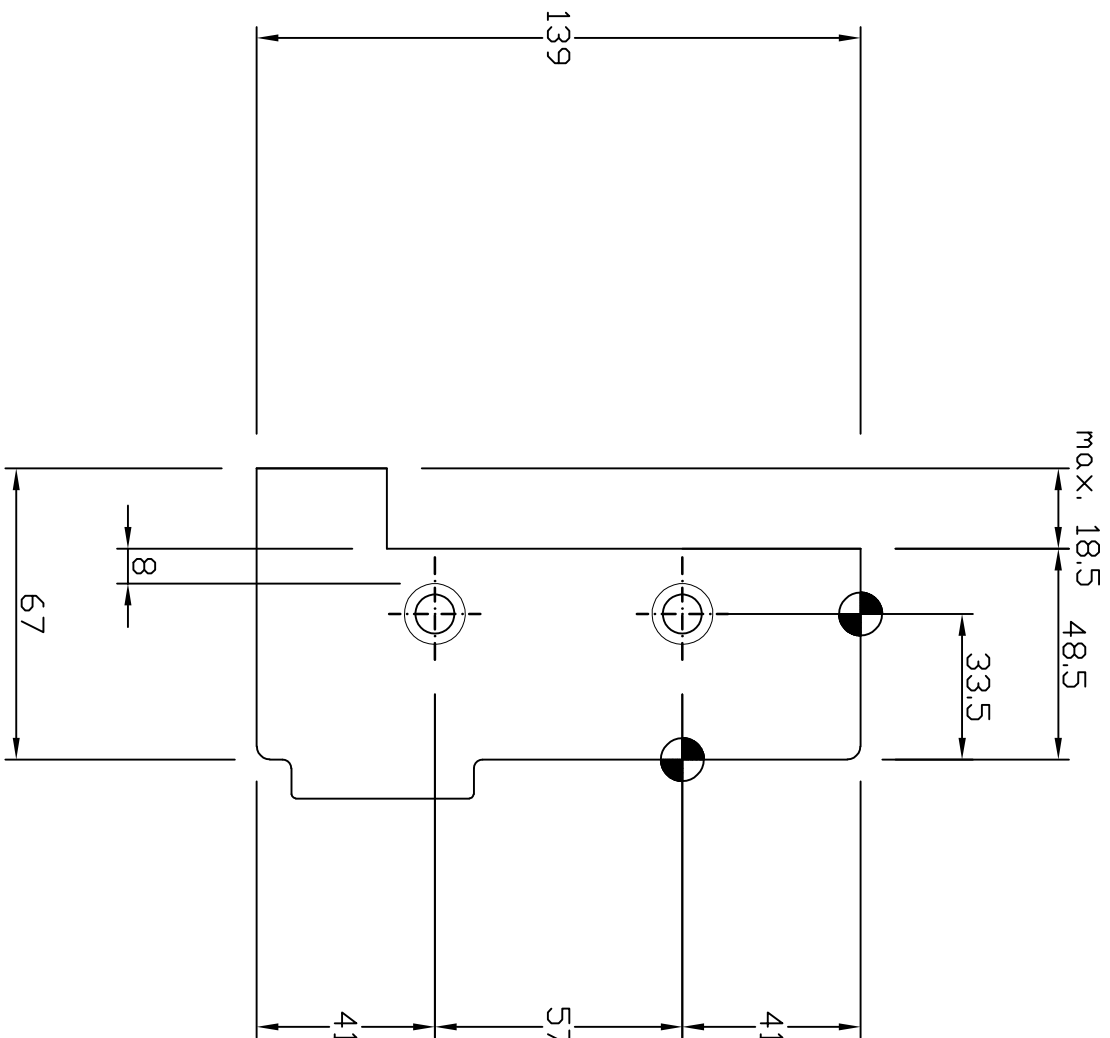
Boorpatroon: HFS33.5 (V139)
