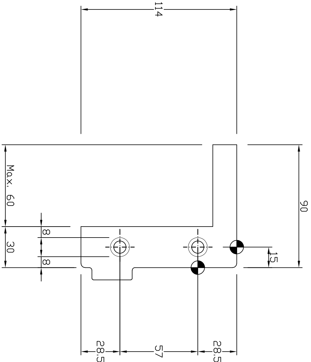
Boorpatroon: HFS15 (V114)
