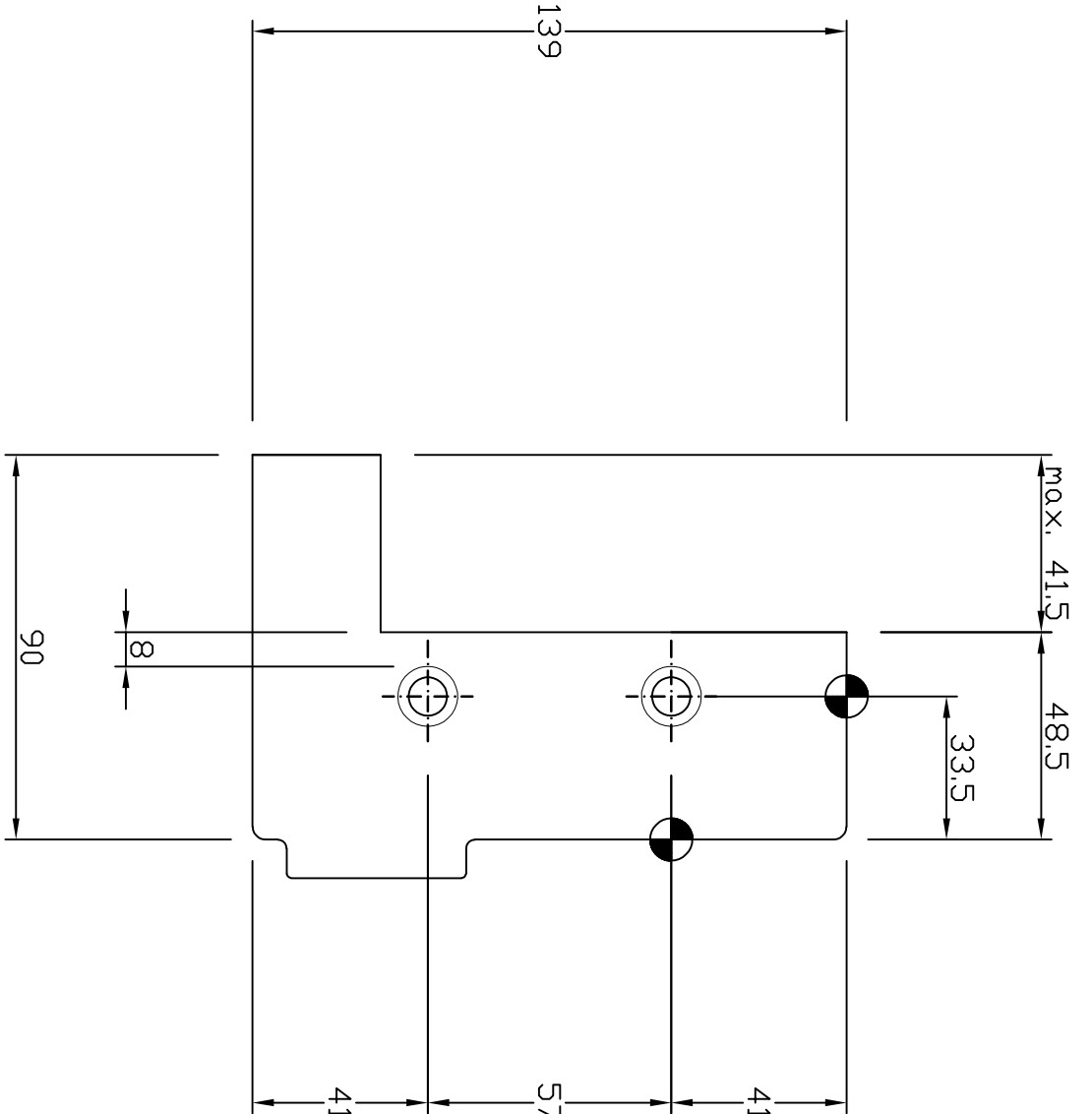
Boorpatroon: HFS33.5 (V139)
