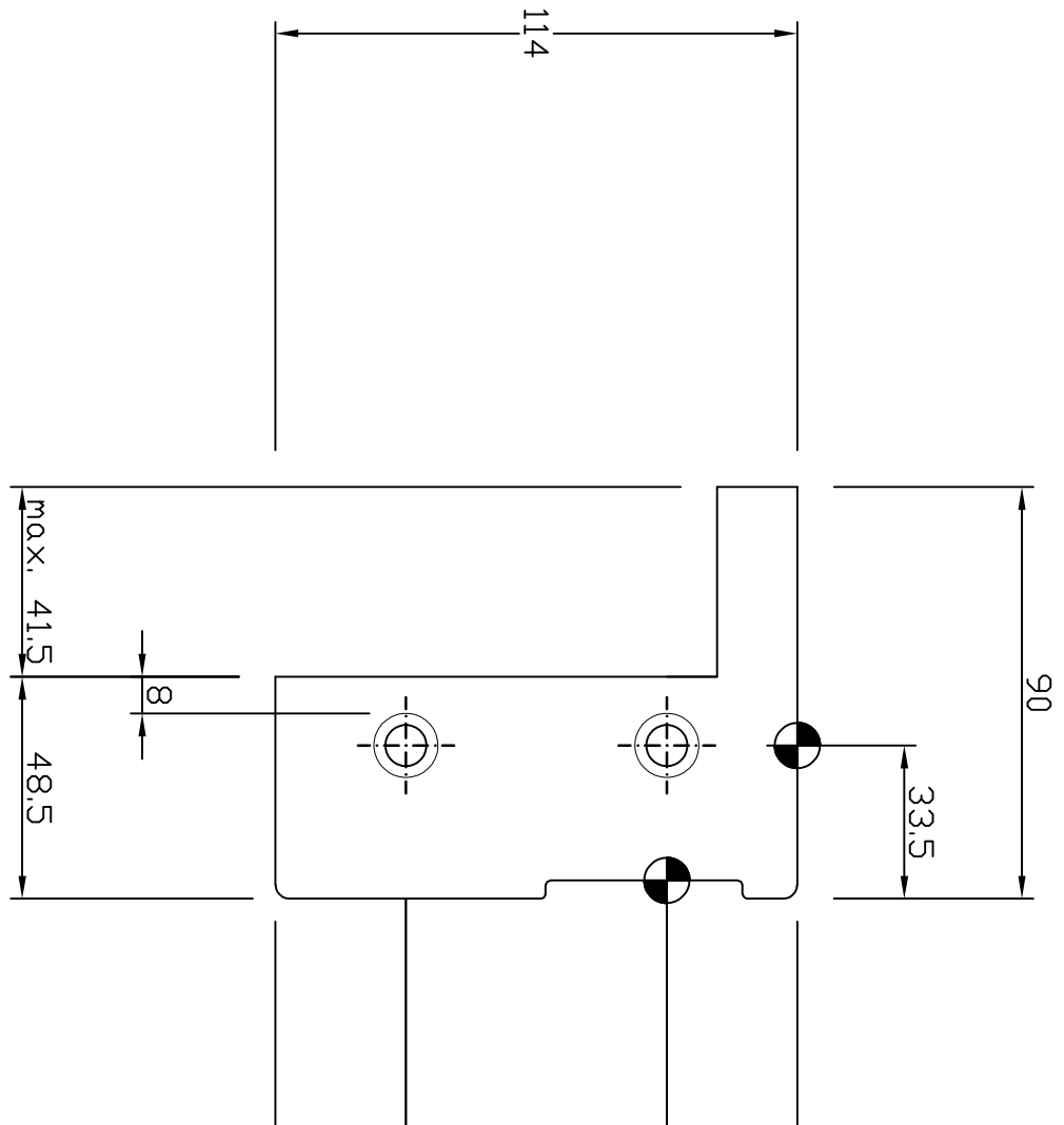
Boorpatroon: HFS33.5 (S114)
