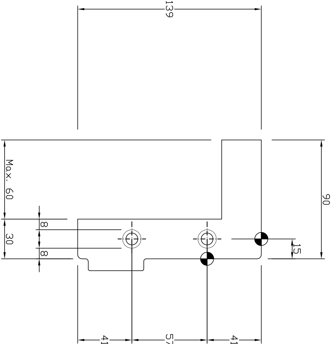
Boorpatroon: HFS15 (V139)
