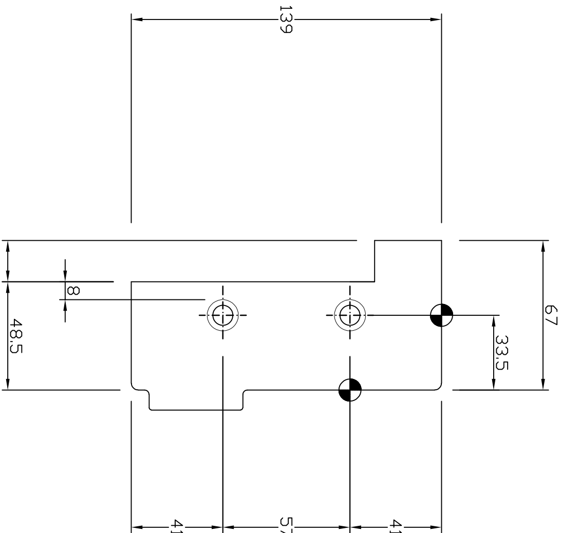
Boorpatroon: HFS33.5 (V139)
