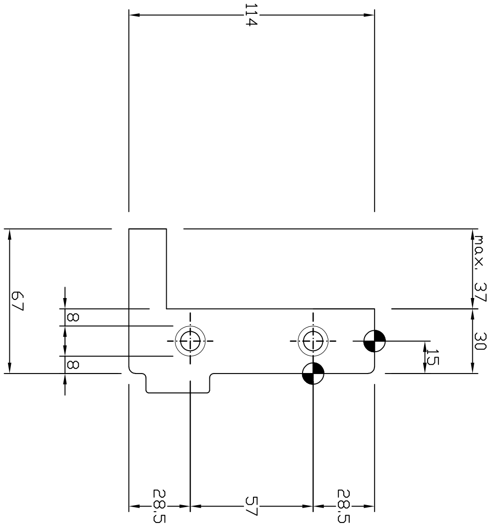
Boorpatroon: HFS15 (V114)
