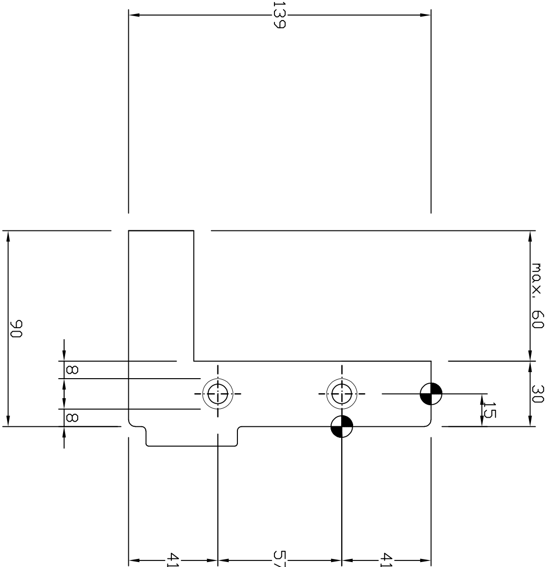
Boorpatroon: HFS15 (V139)
