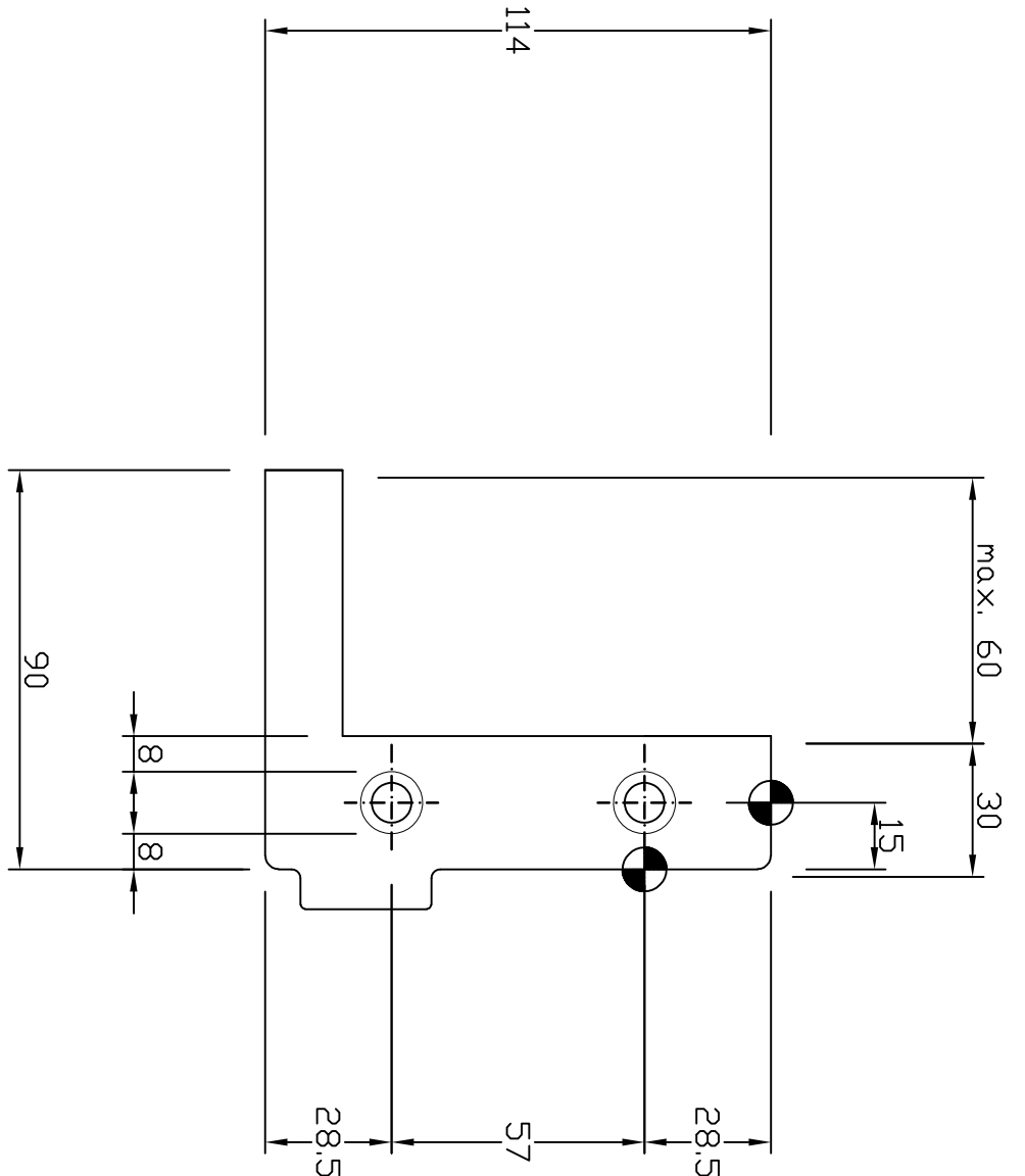
Boorpatroon: HFS15 (V114)
