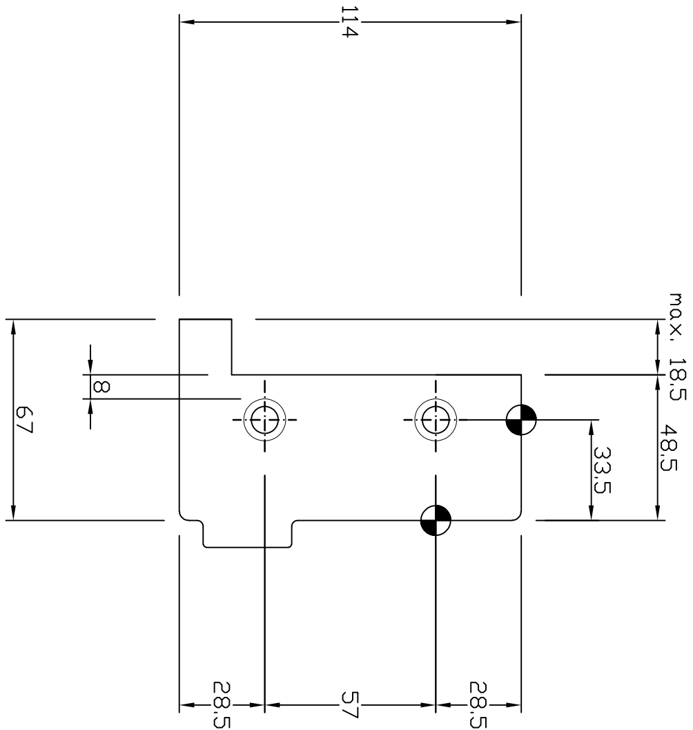
Boorpatroon: HFS33.5 (V114)
