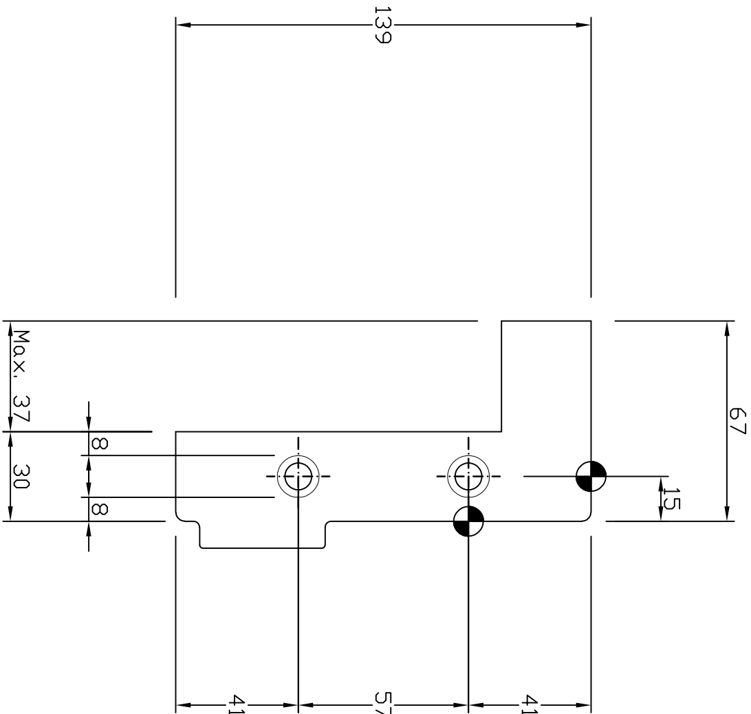
Boorpatroon: HFS15 (V139)
