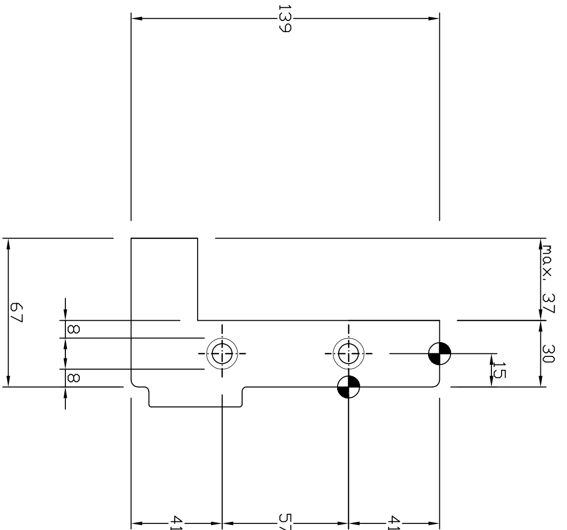
Boorpatroon: HFS15 (V139)
